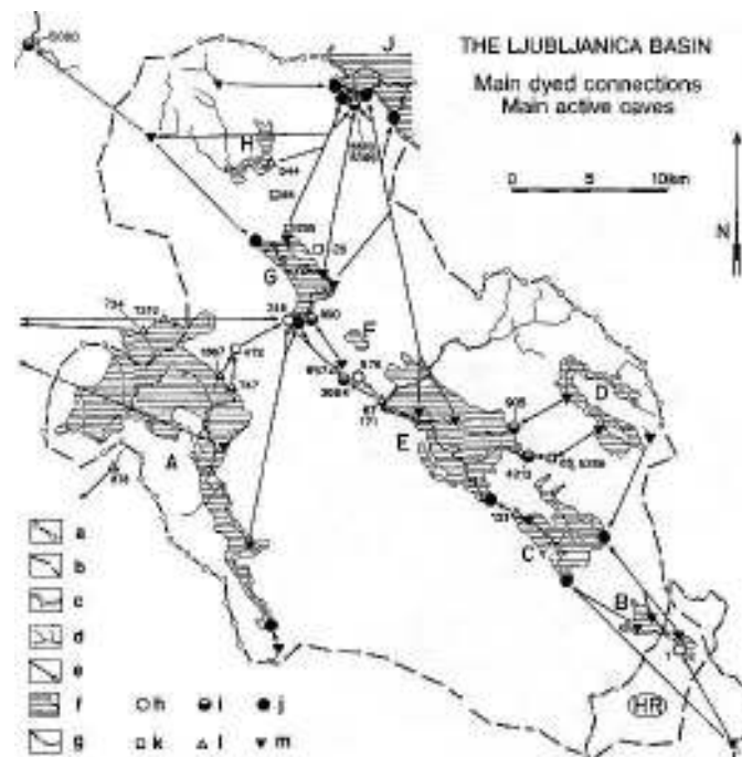
Fig. 3. The Ljubljana Basin.
