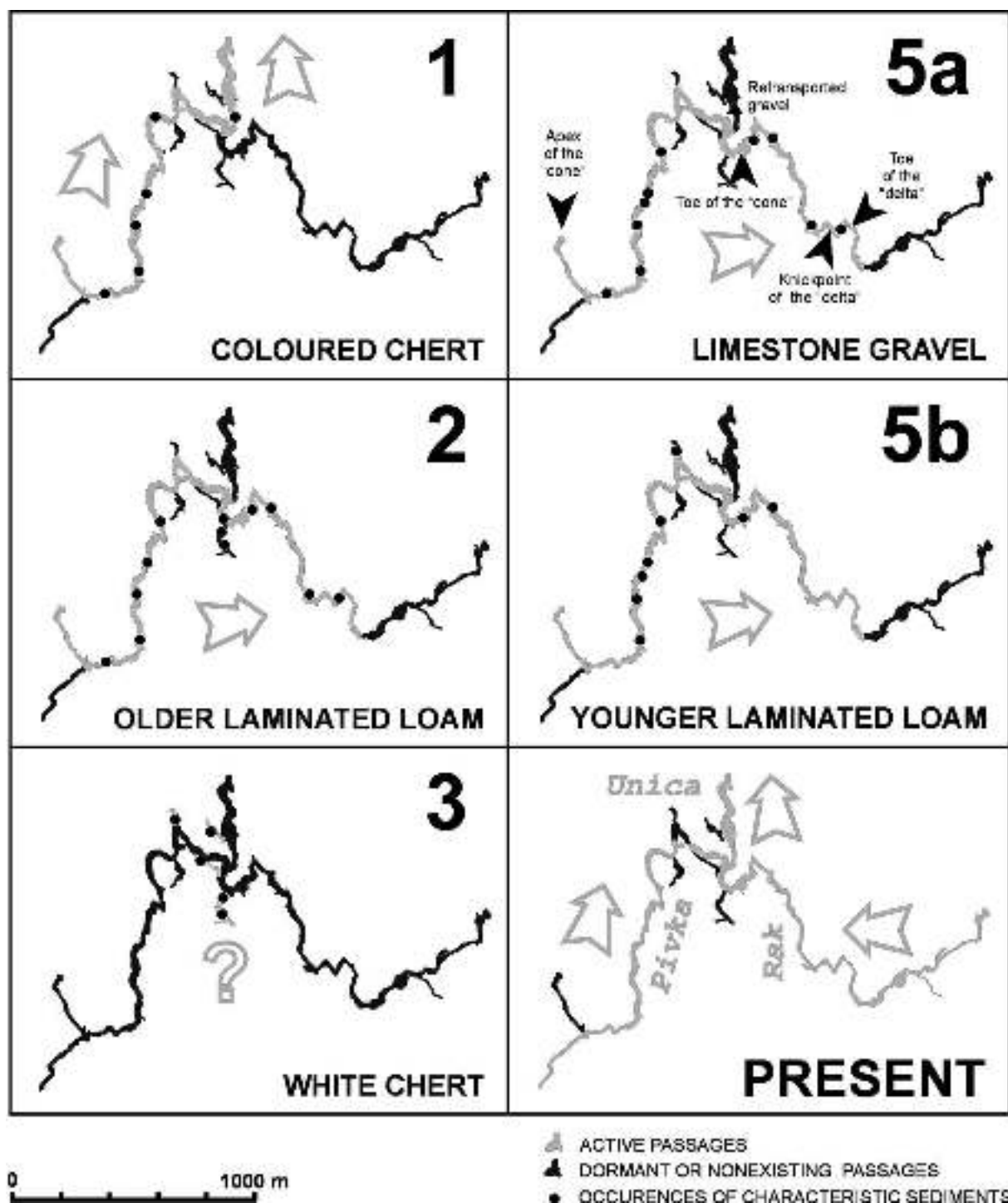
Fig. 12. Zelške jame cave system
