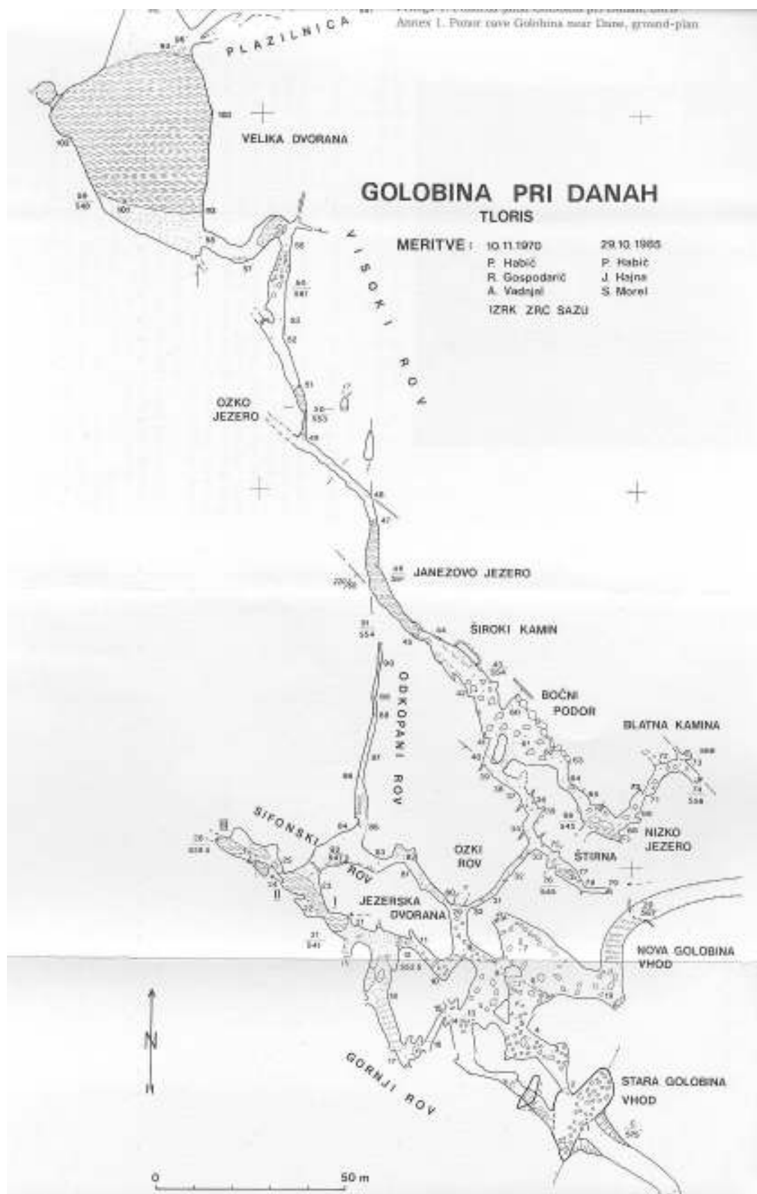
Fig. 8. Golobina pri Danah cave
